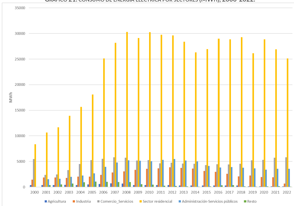
GRÁFICO 21. CONSUMO DE ENERGÍA ELÉCTRICA POR SECTORES (MWh), 2000-2022.
