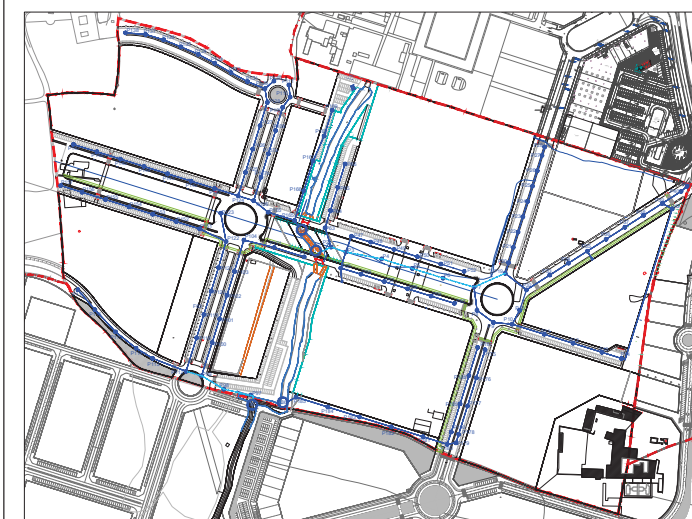
PLANTA GENERAL. E:1/2500
