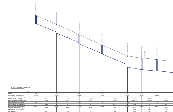
ROTONDA 2 - FINAL AVDA D1
